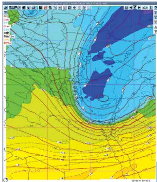
حركة الضغط الجوي ومسار الرياح في اثناء العاصفة "زينة".
